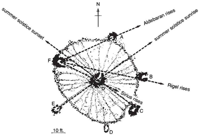
Der Sommeranfang-Steinkreis des Big Horn Medizinrades Wyoming (John A. Eddy, Native American Astronomy, Ausgabe Aveni)
